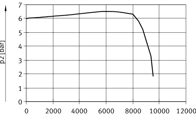
MS6-LRP-1/2-PE10/PI10
